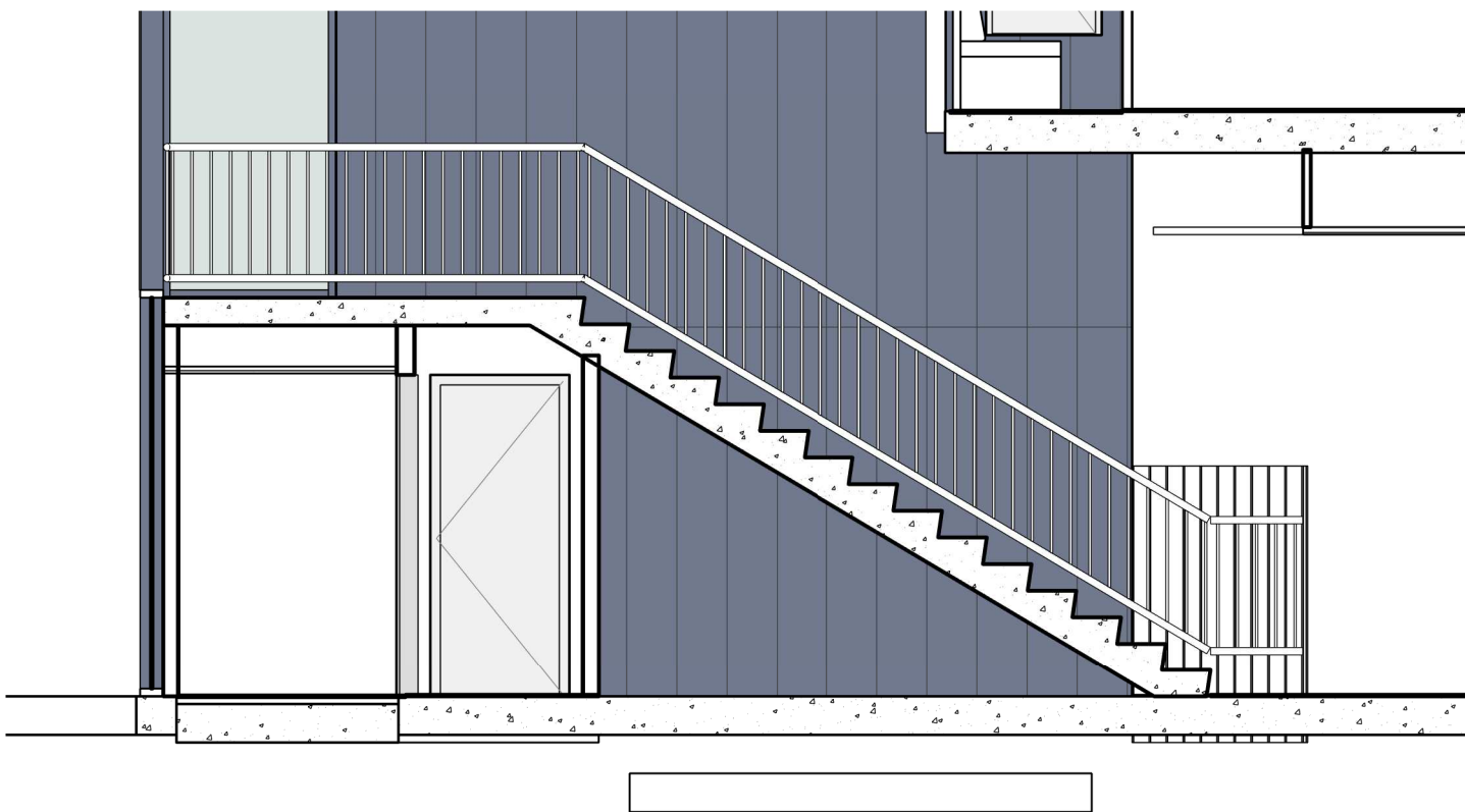
3 Section 14 42-02 1 : 50
