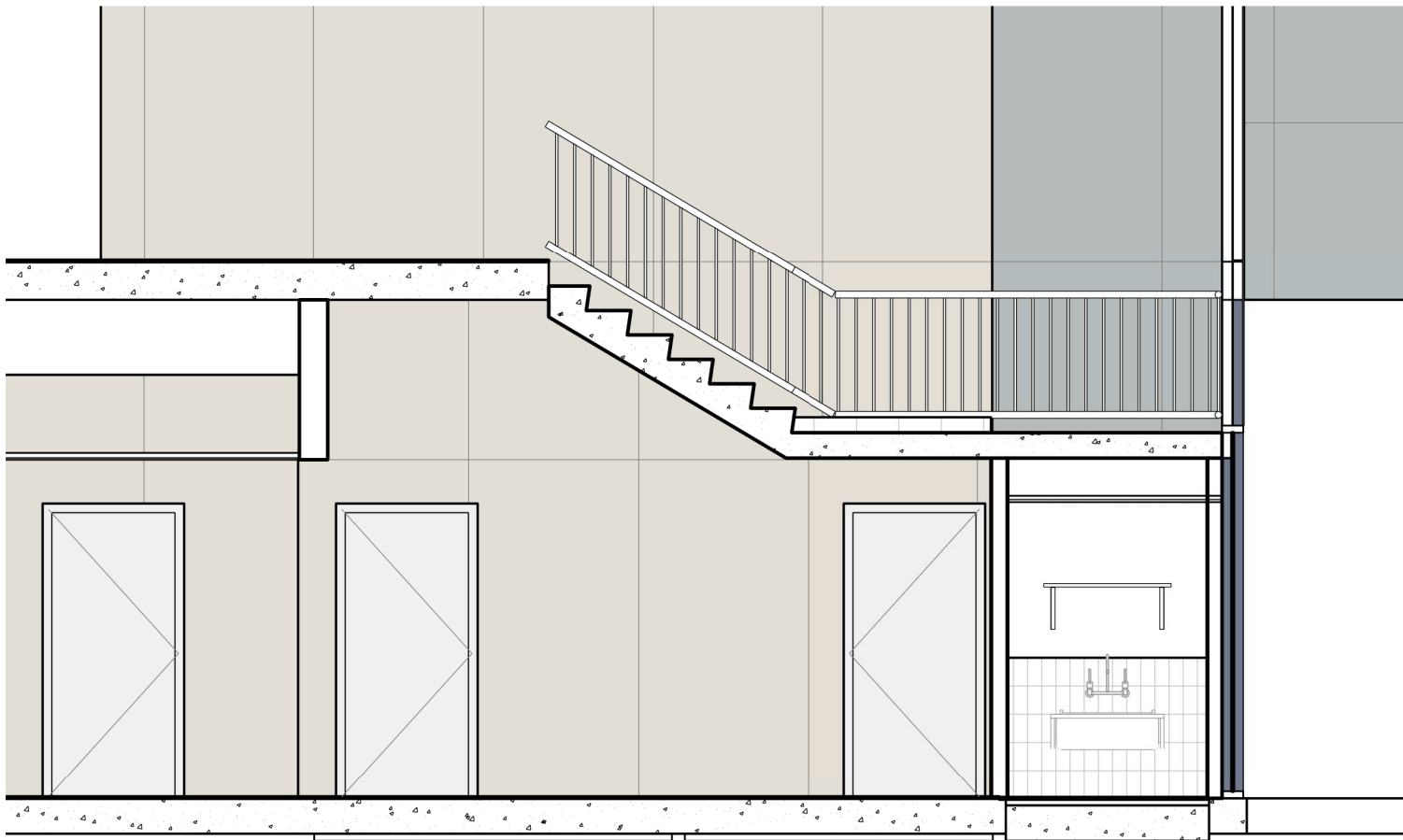
4 Section 15 42-02 1 : 50
